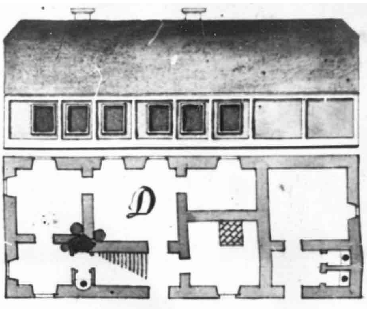
Pálóczi Horváth Ádám füredi kisebbik házának alaprajza
